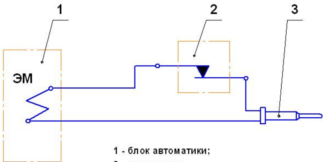
Рис.3 Схема электрическая
