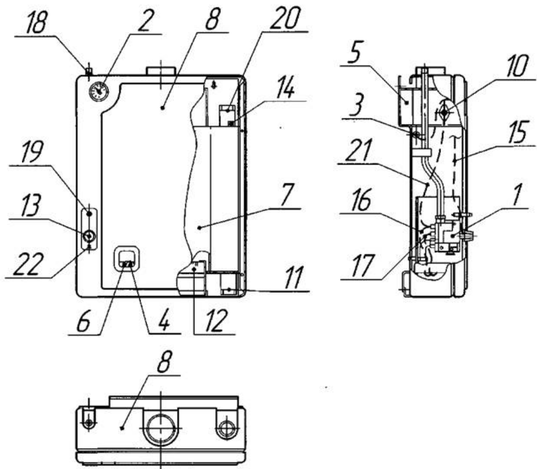
Рис. 1 Конструкция котла
